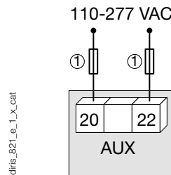
1. Предохранители 0,5 А gG / 0,5 А класса CC.
