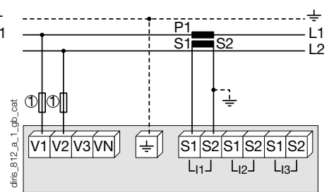
1. Предохранители 0,5 А gG / 0,5 А класса CC.
