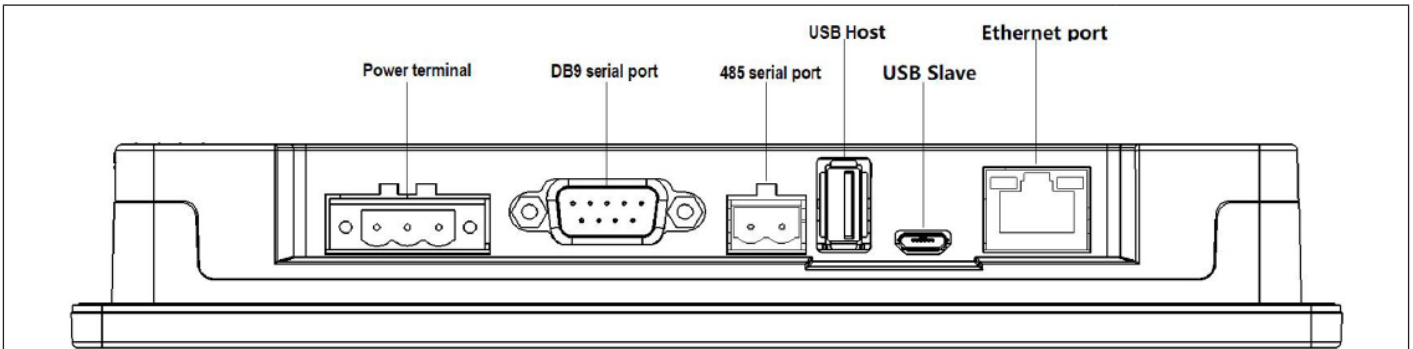
Клеммы подключения питания (Pin1 ~ 3 слева направо)
