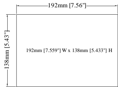
Cutout Dimensions
